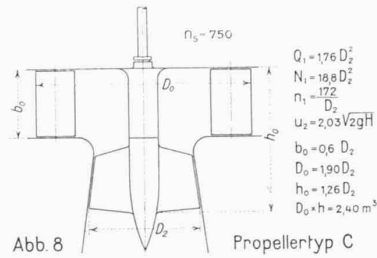
Abb. 8 Propellertyp C
