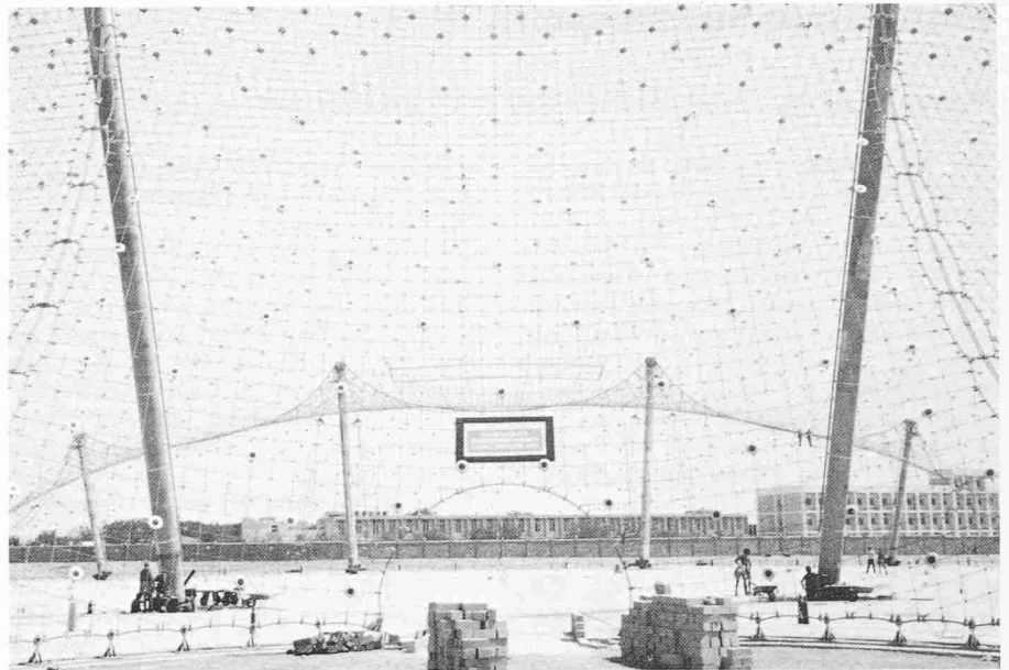
Fertig gespanntes Seiltragnetz mit montierten Membranteilern
