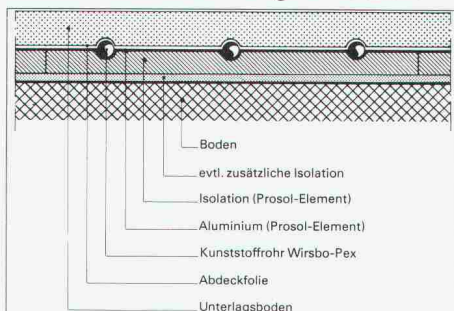
Herkömmliches Bodenheizungssystem
