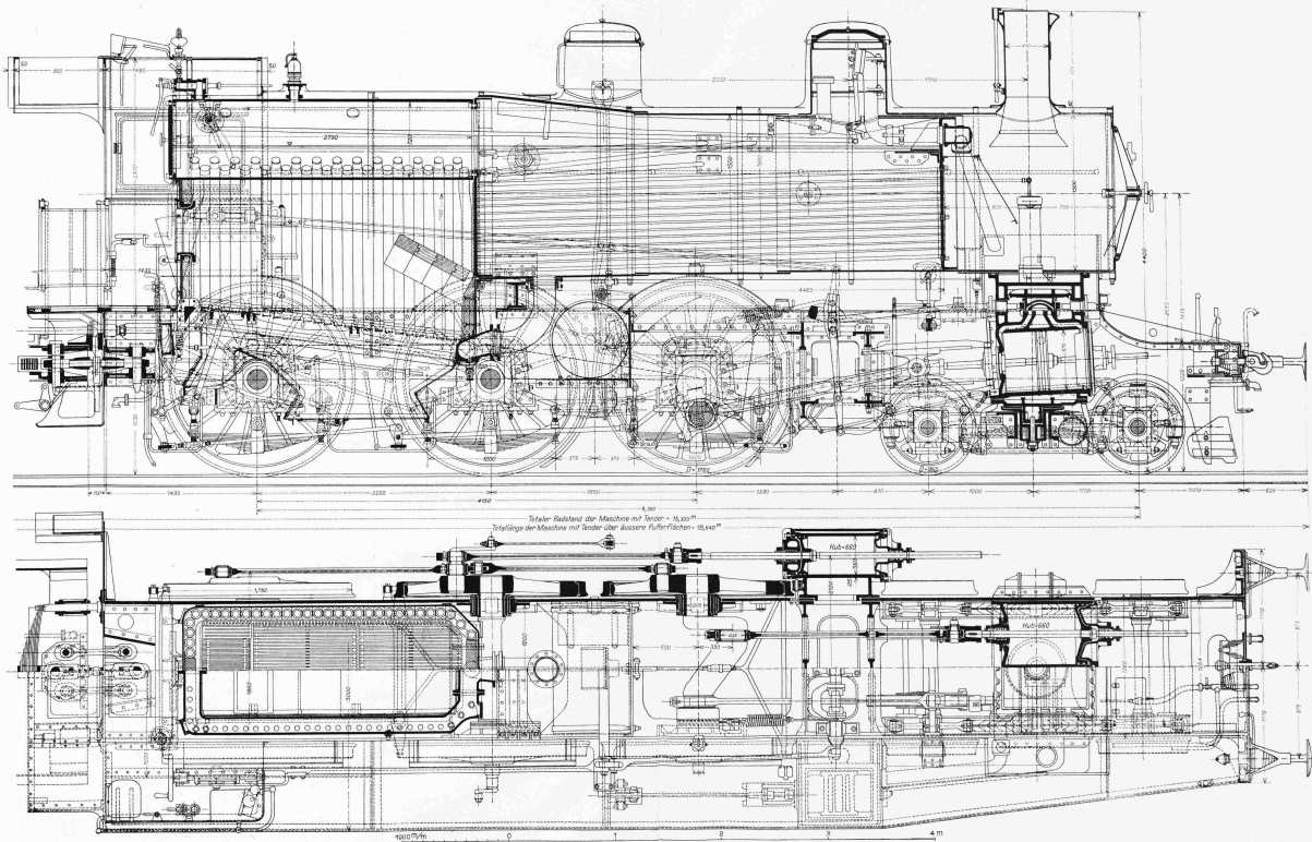
Längs- und Horizontalschnitte. — Masstab 1:35.
