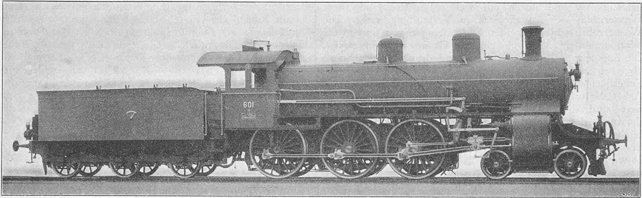
Abb. 5. A 3 / 5 Heissdampf-Vierzylinder-Verbund-Lokomotive gebaut von der Schweiz. Lokomotiv- und Maschinenfabrik Winterthur.
