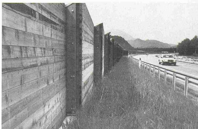
Die absorbierende Version mit eingelegtem Schallschutzmaterial im Seeland (Photo: Renfer, Biel)
