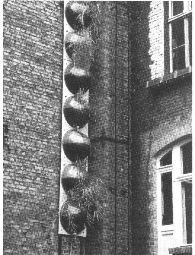
Vertikalsumpf im Altbau: In den Behältern wachsen Schilf und Binsen als Substrat dient Blähton. Das Grauwasser wird in den obersten Behältern gepumpt und fließt im freien Fall von einem zum nächsten nach unten.
