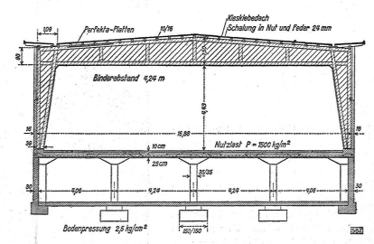
Abb. 7 Querschnitt 1:200 mit Fichte für 1,5 t pro m² Nutzlast über Kellergeschoß und genagelte Rahmenbinder über Erdgeschoß. Spannweite ca. 17 m, Binderabstand 4,2 m
