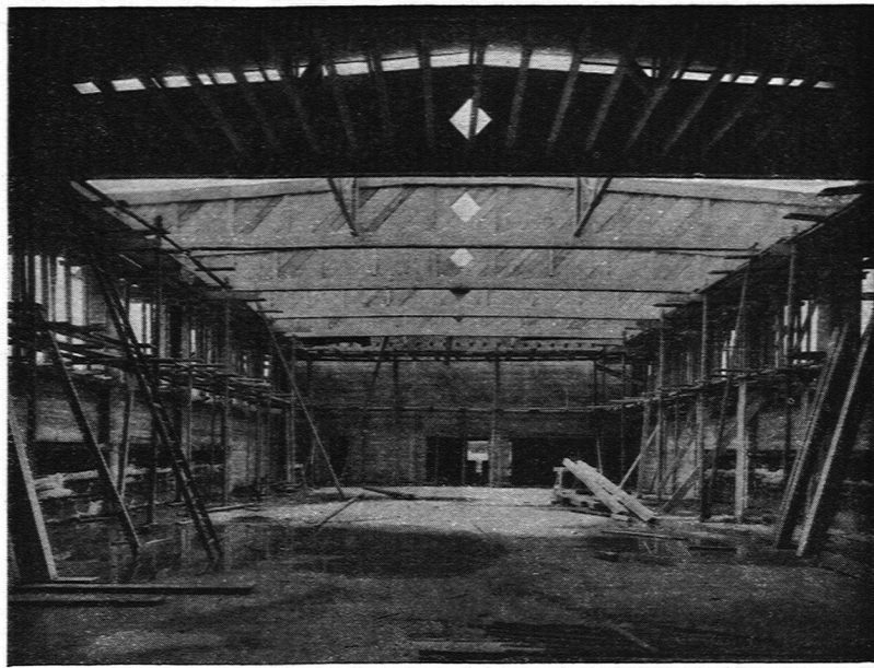
Abb. 1 Turnhalle der Kantonsschule Solothurn mit aufgerichteten Nagelbindern
