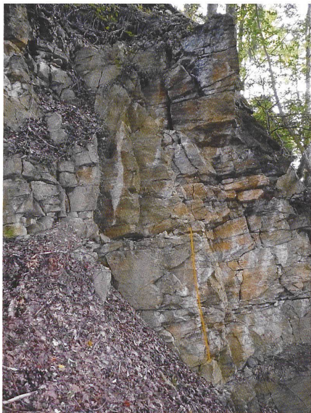
Fig. 7: Aufschluss 2 bei der Lokalität Ängistein. Schräg geschichtete Kalkarenite des Ängistein-Members. Die Foreset-Beds der Schrägschichtung weisen einheitlich auf eine Schüttung nach Süden. Die Kalke bilden eine markante Geländekante.
