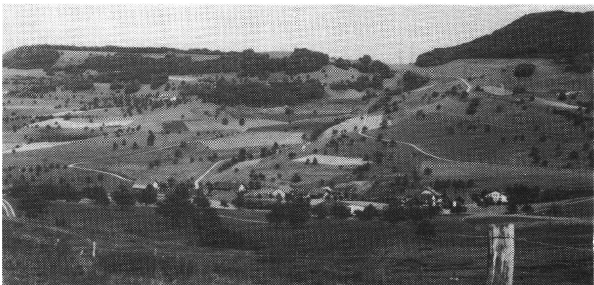
Abb. 8: Mandacher Aufschiebung. Blick gegen E über Büren auf Laubberg links (N) und Bürerhorn rechts (S), im Sattel dazwischen die Mandacher Störung, an der Keuper, Lias, Opalinus-Ton und Dogger des Bürerhorns gegen den schwach S-fallenden Haupttrogenstein des Laubbergs aufgeschoben sind. Foto PBB: 10.7.85
