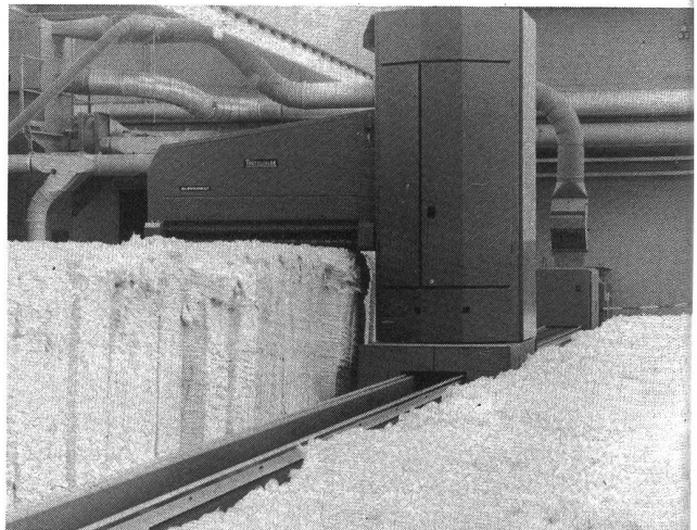
In der Spinnerei-Vorbereitung ist ein automatischer Ballenöffner Blendomat der Firma Trützschler eingesetzt.
