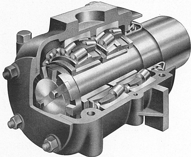
Achsbüchse mit Pendelrollenlagern
