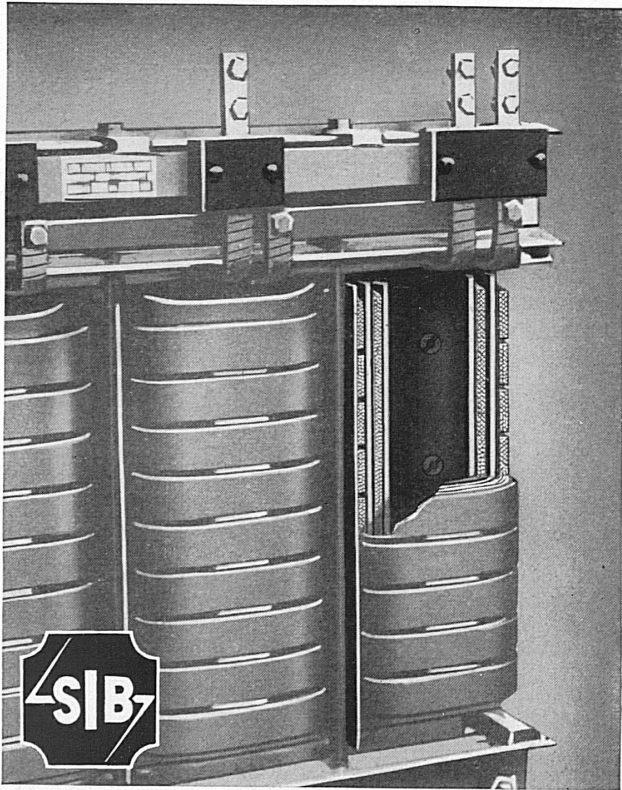
Spezialitäten für Transformatoren: Wicklungsdrähte, Imprägnier- und Decklacke, Isolierstücke aus Dellit-Hartpapier, Isolierbänder
