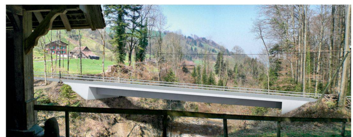
07 «Nepomuk»: Einfach, schnörkellos und funktional – Stahl-Beton-Verbundbrücke mit zwei Längsträgern und leichter Rahmenwirkung
