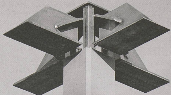
Stützenkopfverstärkung T-WALM®
