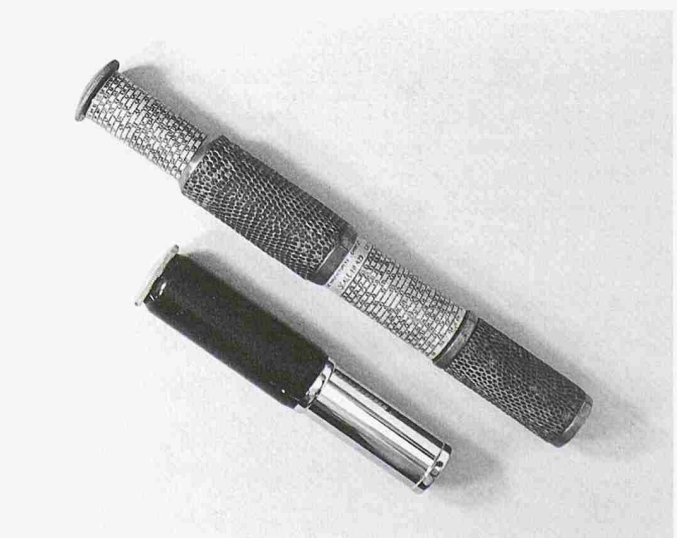
8 Englischer Rechenzylinder «Otis King», teleskopisch zusammenschiebbar für die Tasche, mit schraubenlinienförmigen Skalen von fast 1,7 m Länge (66") bei einer Baulänge von nur 15 cm, bzw. ausgezogen 26 cm. Die «Otis King» wurden von der Carbic Ltd., Coventry, später London, gebaut. Um den unterschiedlichen Wünschen bezüglich Skalen zu entsprechen, konnte aus 13 Typen ausgewählt werden. Das zusammengeschobene Objekt (ca. 1960) ist verchromt und mit Boxcalf, das andere, ältere (ca. 1930), besteht aus Messing und ist mit Schlangenleder bezogen
