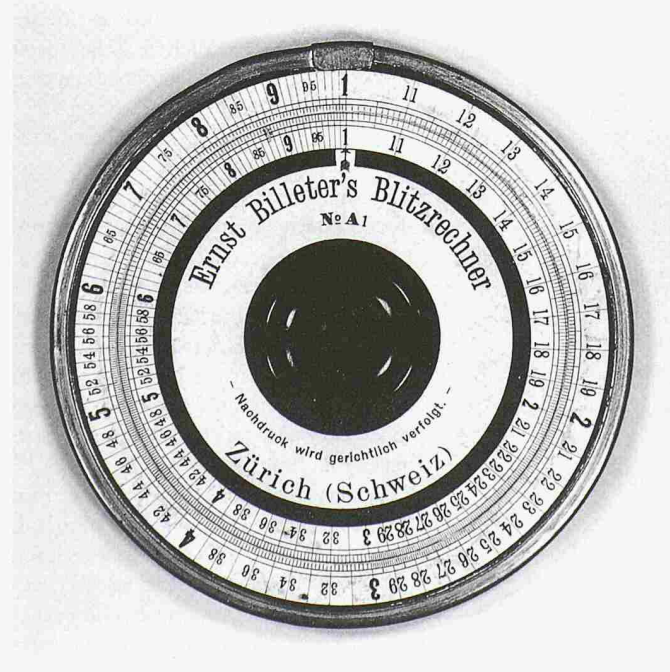
7 Rechenscheibe «Blitzrechner» von Ernst Billeter, Zürich, um 1912. Die Typenbezeichnung A1 kennzeichnet die Scheibe mit einer Skalenlänge von 30 cm; daneben gab es noch ein Modell A2 mit einer solchen von 75 cm
