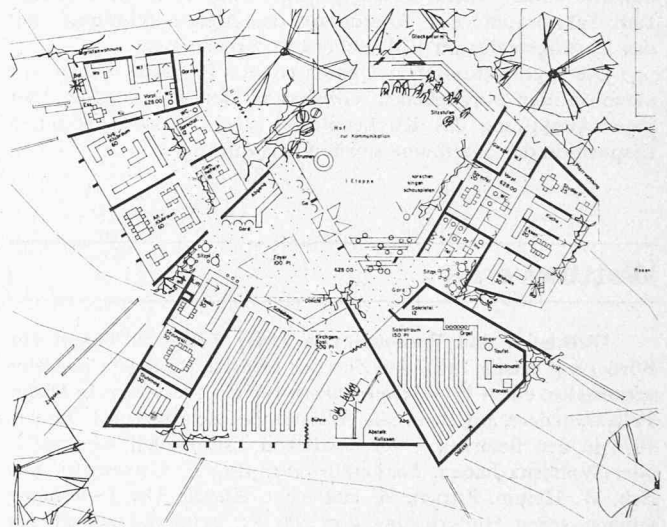
Grundriss Eingangsgeschoss 1:800
