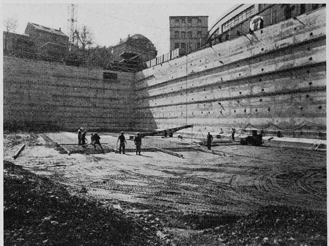
Bild 3. Nach der Unterfangungsmethode erstellte Baugrube der Parkgarage Elisabethenschanze in Basel. Die einzelnen Elemente sind mit Kiesankern zurückverankert
