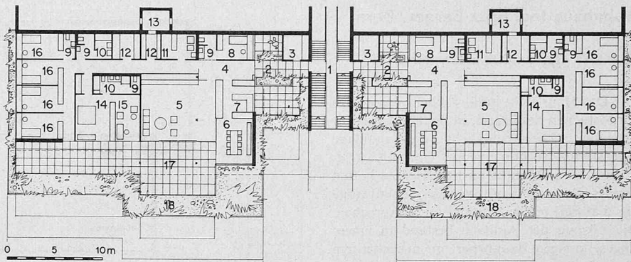
Grundriss. Terrassengeschoß 1:600. Legende: 1 Treppenhaus mit Schräglift, 2 Vorhof, 3 Réduit, 4 Entrée, 5 Wohnraum, 6 Esszimmer, 7 Küche, 8 Arbeitsraum, 9 WC, 10 Bad, 11 Wäscherei, 12 Schrankraum, 13 Klimagerät, 14 Elternzimmer, 15 Studio, 16 Zimmer, 17 Terrasse, teilweise gedeckt, 18 Grünfläche
