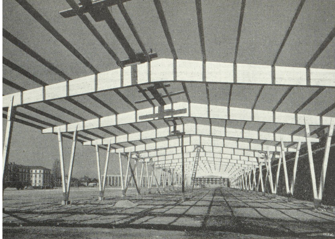
Charpente collée : Halles démontables au Comptoir Suisse.
