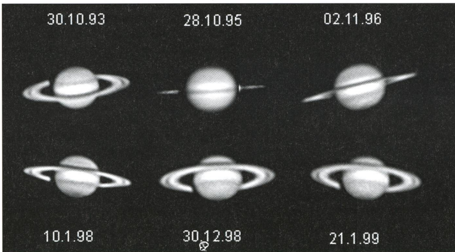
Saturn 1993-1999; Alle Aufnahmen mit CCD Kamera LYNXX2, Cassegrain f=6000\text{mm} , F/D=1:50
