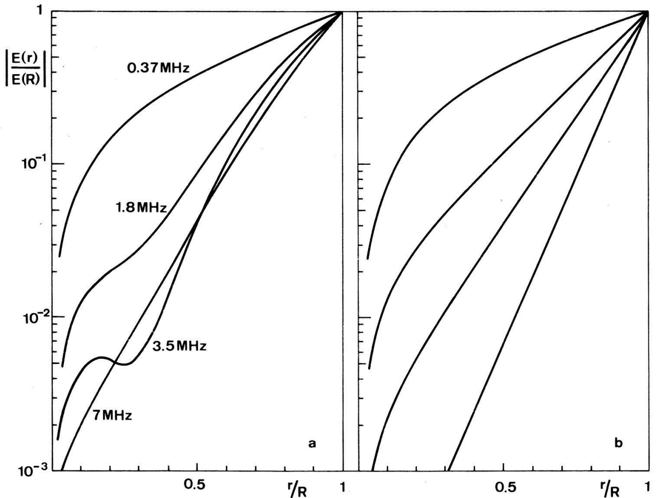
Figure 15 (a) Champ électrique calculé à partir des mesures d'amplitude et de phase pour le plasma 2; (b) Cas normal.
