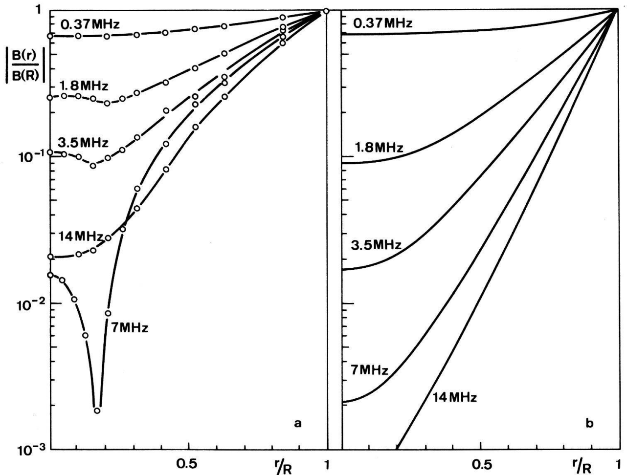
Figure 8 (a) Amplitude du champ magnétique pour le plasma \bar{n}_e = 1.4 \times 10^{12} \text{ cm}^{-3} , T_e = 2 \text{ eV} , \nu = 4.5 \times 10^7 \text{ s}^{-1} ; (b) Cas normal.
