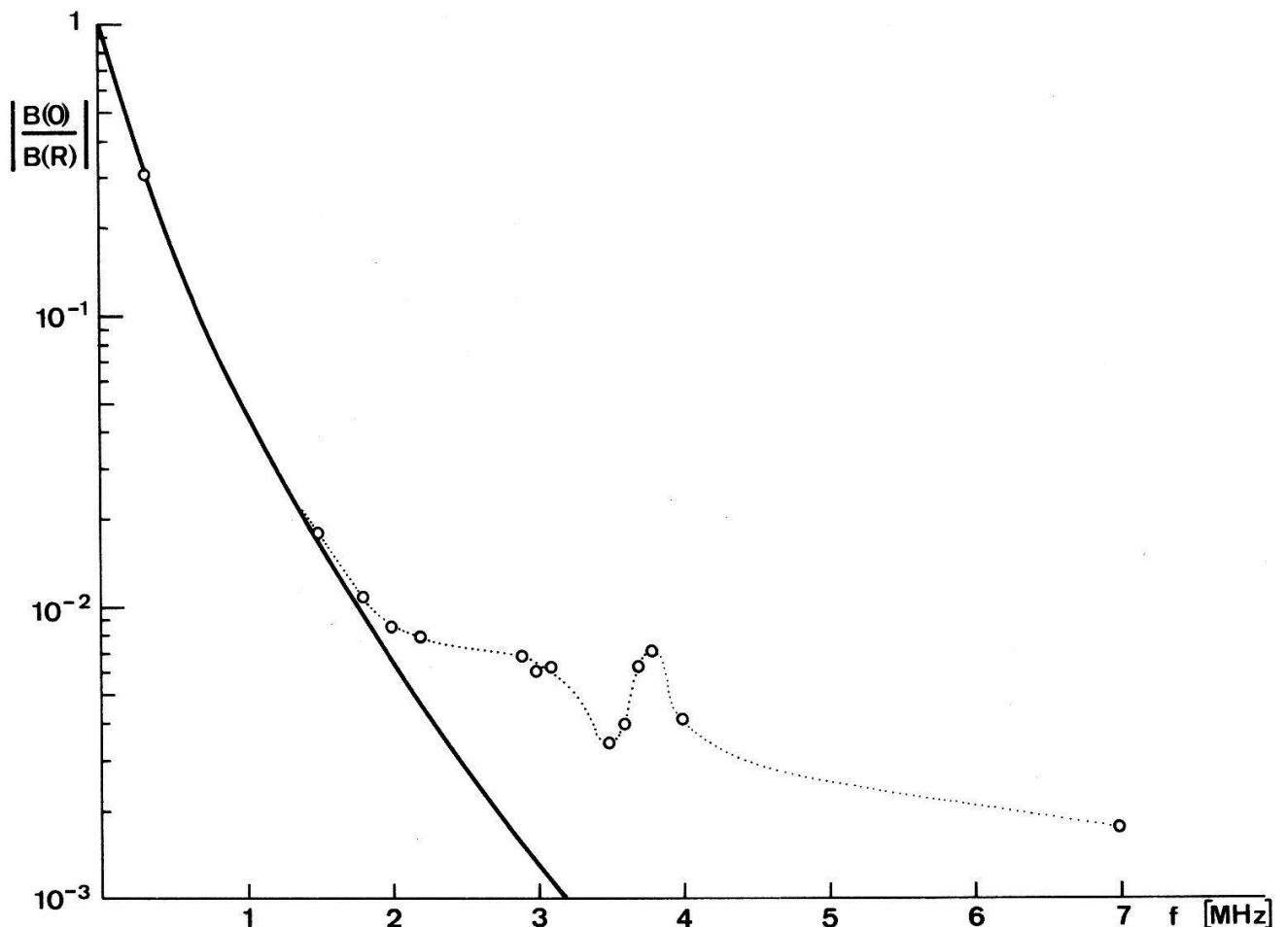
Figure 10 Amplitude du champ sur l'axe en fonction de la fréquence pour le plasma 1.
