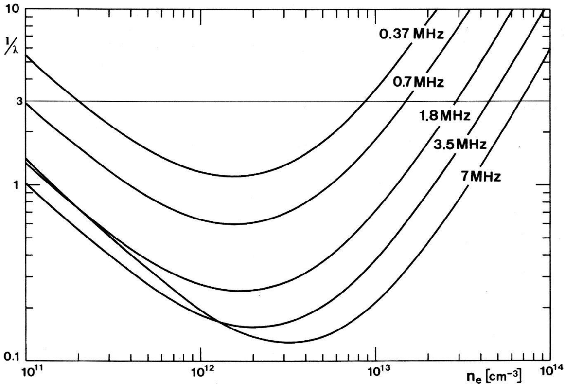
Figure 1 Paramètre d'anomalie 1/\lambda pour un plasma d'argon de 2 eV, et une pression de remplissage de 10 mTorr.
