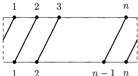
\tau_n: n \rightarrow n
