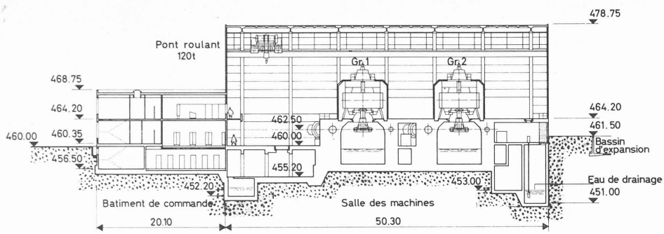
Coupe longitudinale
