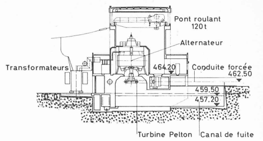
Coupe transversale
