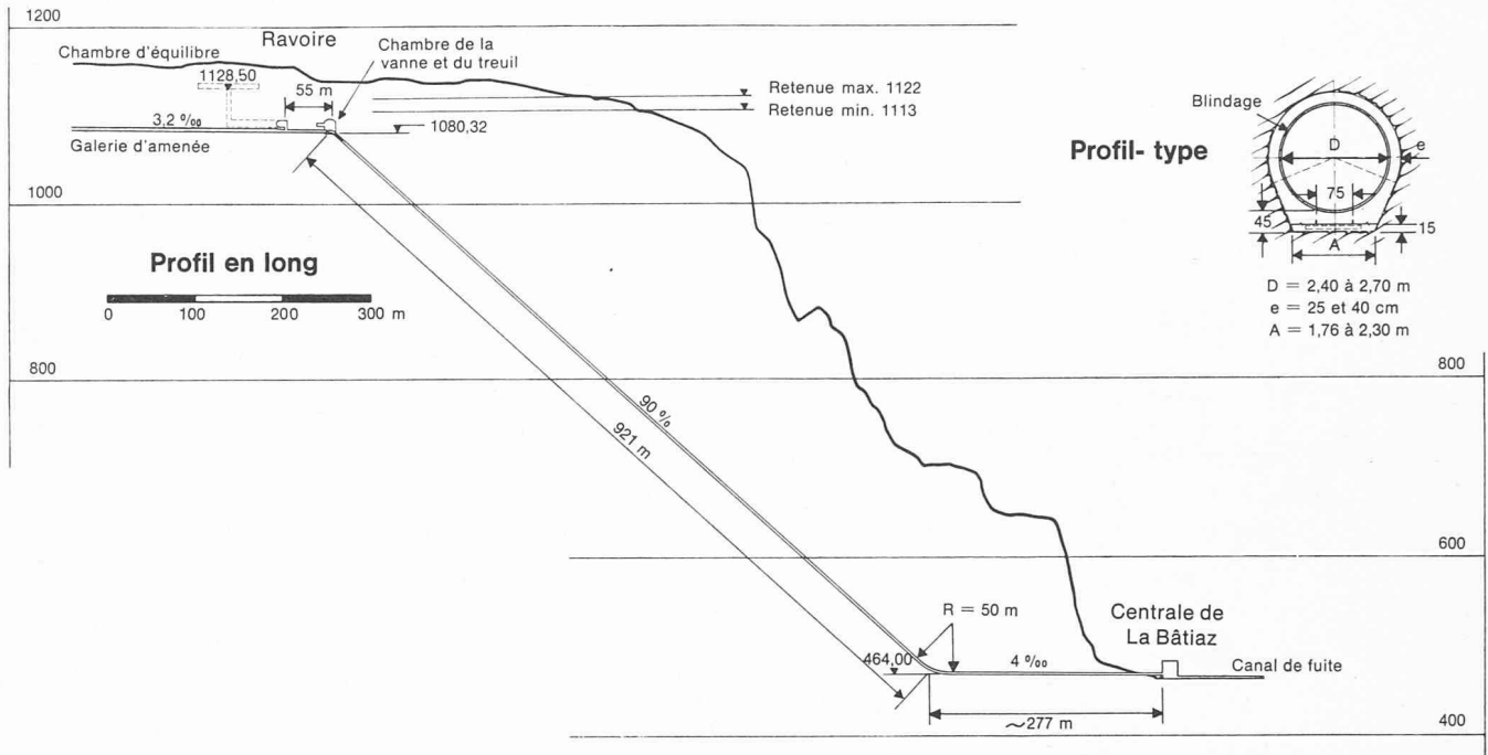
Fig. 16 — Profil en long et profil-type du puits blindé de Ravoire.
