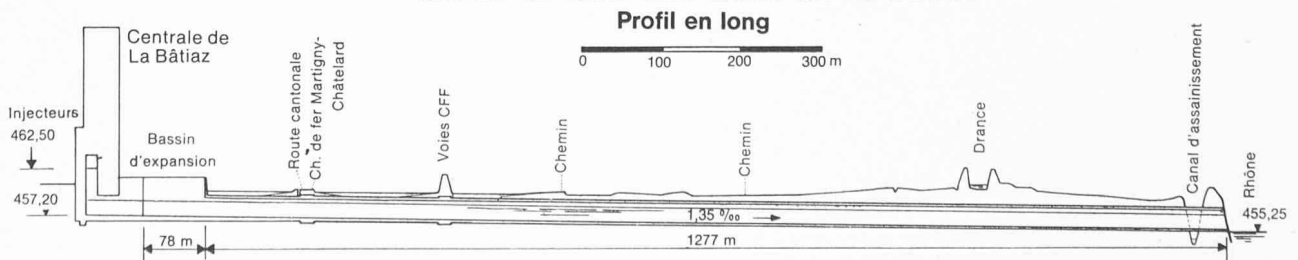
Fig. 18 — Profil en long et profil-type du canal de fuite de La Bâtiáz.
