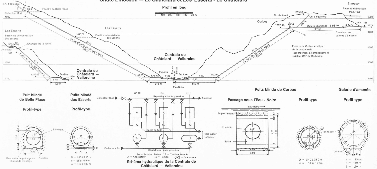
Fig. 13 — Chutes Emosson-Le Châtelard et Les Esserts-Le Châtelard ainsi que le puits blindé de Belle-Place. Profils en long, profils-types et schéma hydraulique de l'usine de Châtelard-Vallorcine.
