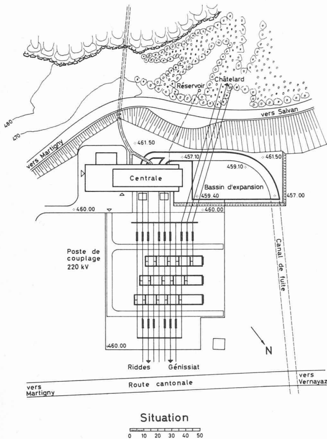
Fig. 17 — Situation de la centrale de La Bâtiáz.
