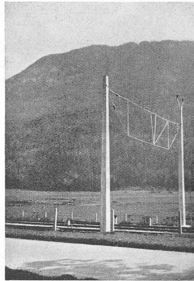
Fig. 13. — Vue d'un pylône de la ligne Auvernier-Les Verrières.
