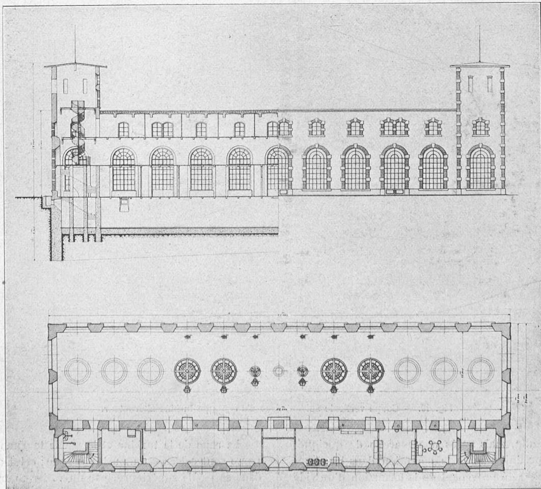
Fig. 18. — Plan et coupe de l'usine. — Echelle : 1 : 500.
