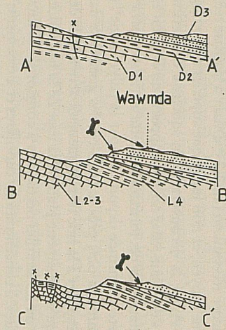
Fig. 8 Carte géologique de la cuvette de Tilougguit; coupes géologiques schématiques dans la partie septentrionale, montrant la relative concordance des «Couches rouges» (coupe A-A'), puis leur nette discordance sur un substratum basculé (coupes B-B' et C-C'). Coordonnées Lambert Nord-Maroc.
